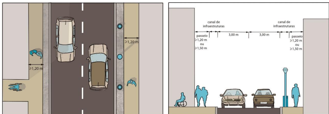
Figura 5. Exemplo perfil-tipo 5
