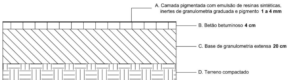
Figura 53. Perfil transversal tipo – pavimento betuminoso com revestimento slurry
