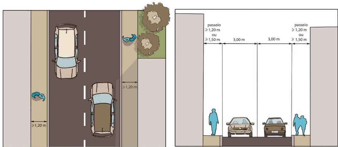
Figura 4. Exemplo perfil-tipo 4
