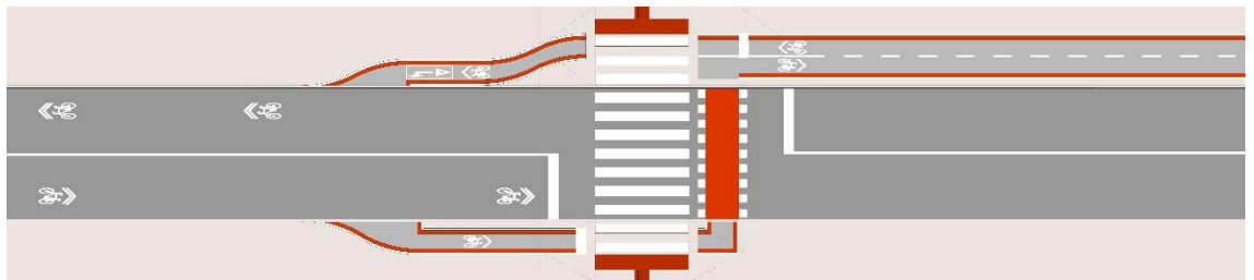
Figura 39. Transição de pista ciclável bidirecional para ciclovia partilhada na via
