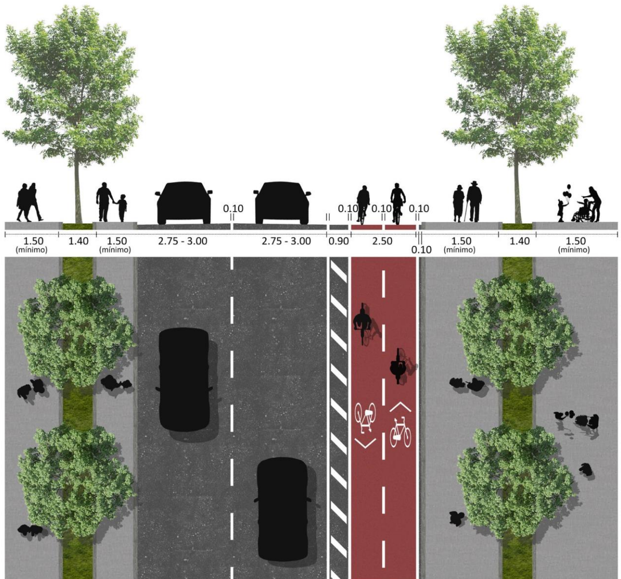
Figura 26. Perfil-tipo de corredor ciclável bidirecional
