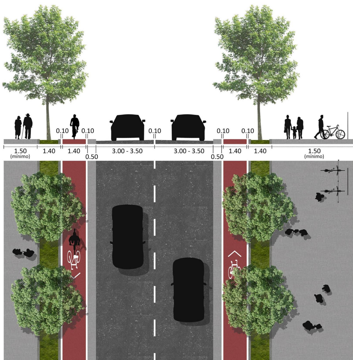
Figura 24. Perfil-tipo de pista ciclável unidirecional
