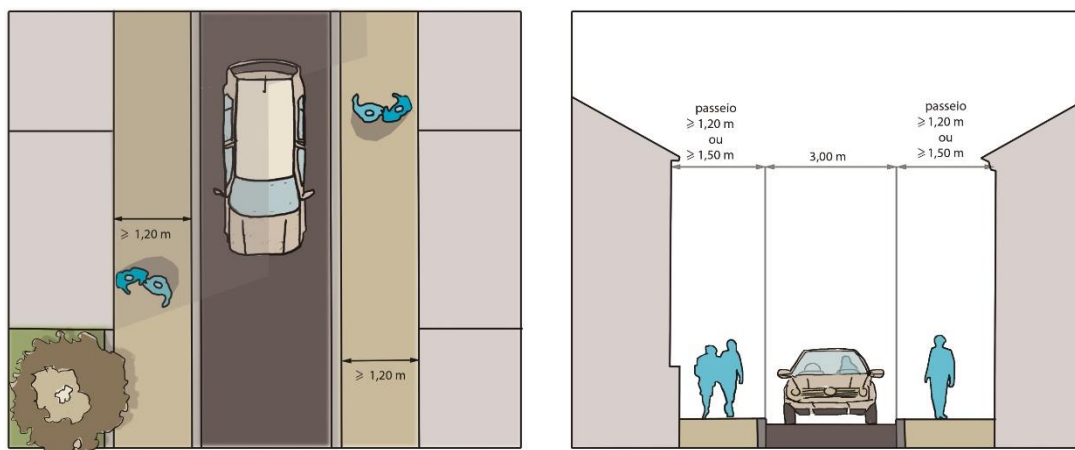
Figura 3. Exemplo Perfil-tipo 3
