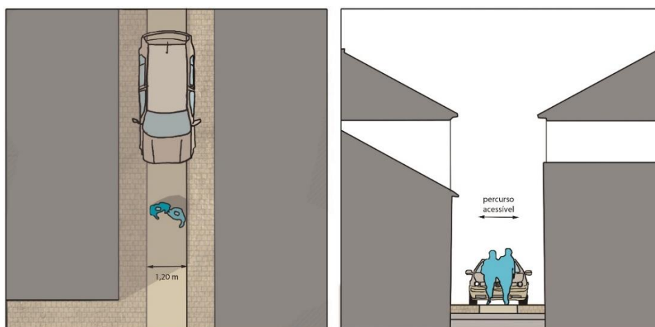
Figura 1. Exemplo perfil-tipo 1
