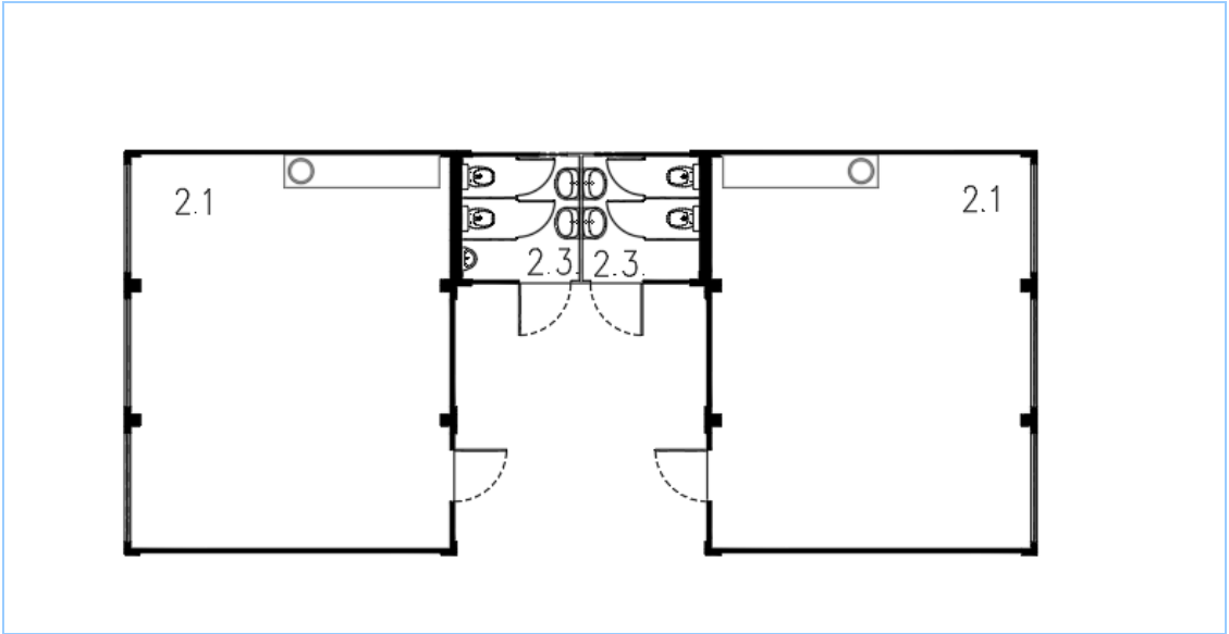
Planta do monobloco
