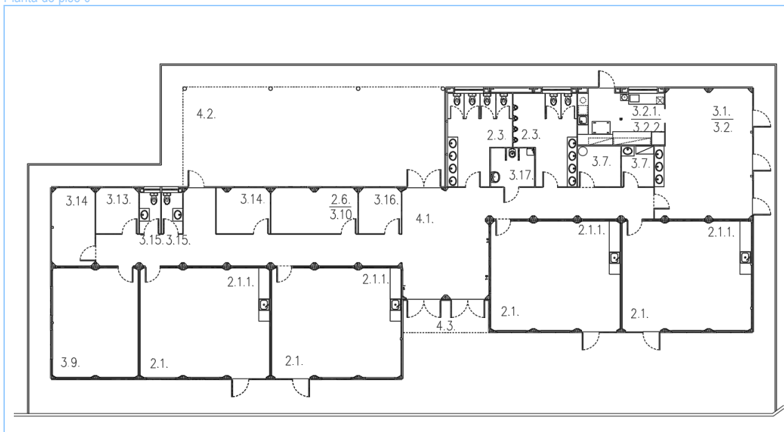
Planta do piso 0
