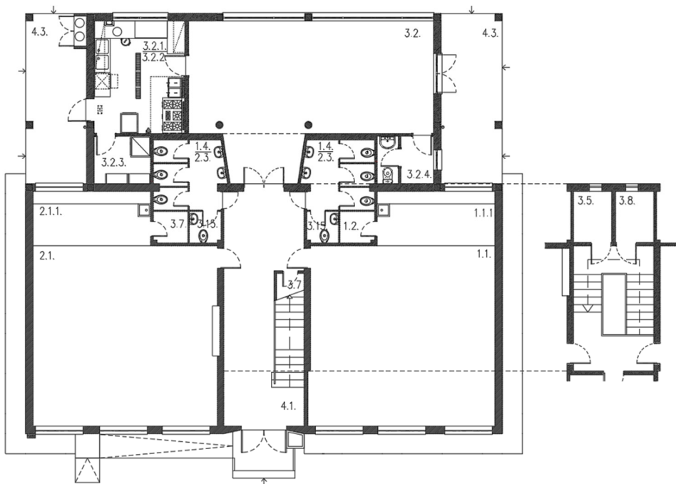
Planta do piso 0 e piso intermédio
