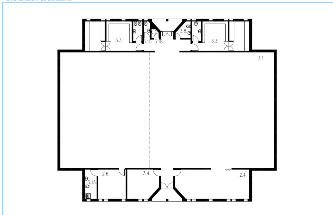
Planta do piso 0 do polivalente
