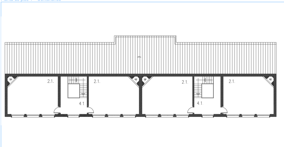
Planta do piso 1 – Centenários
