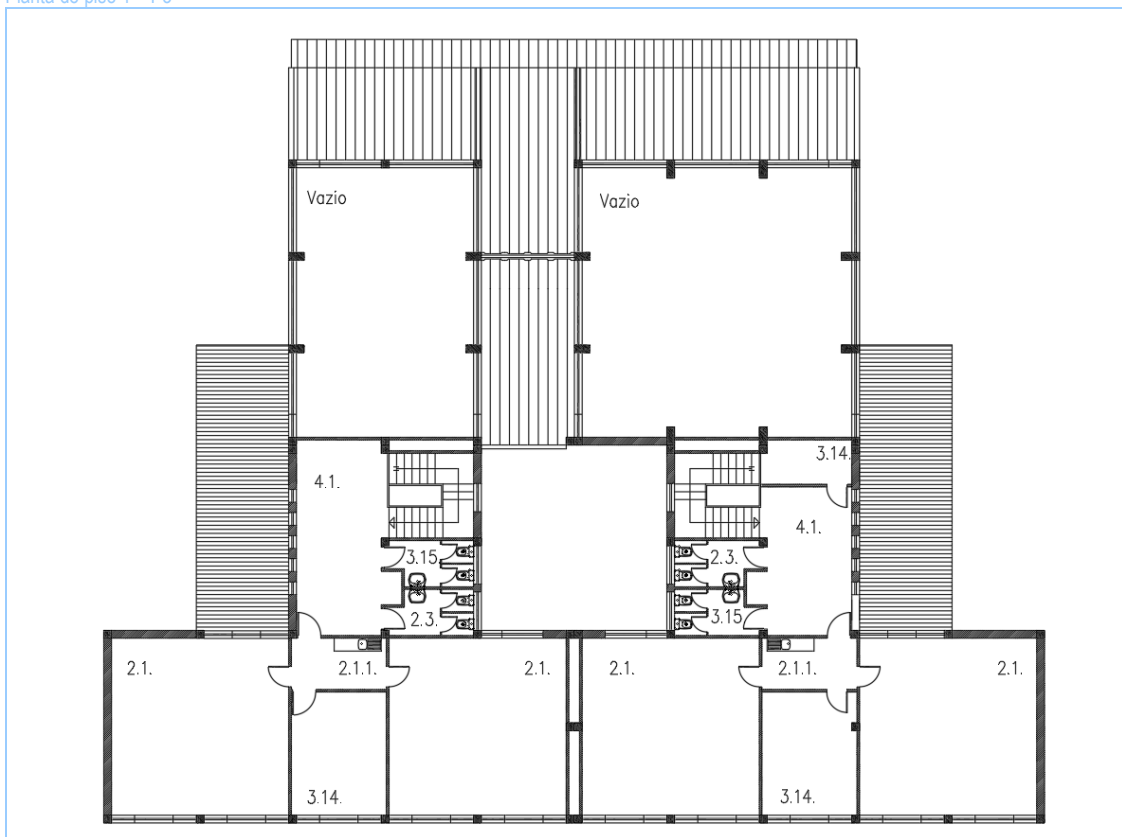
Planta do piso 1 – P3
