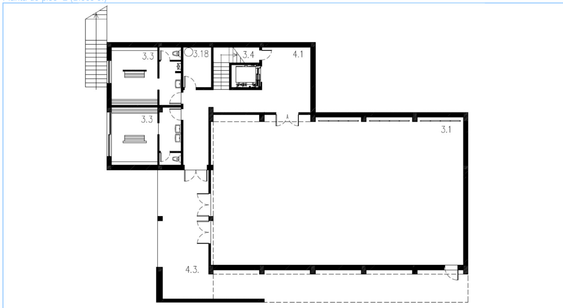
Planta do piso -2 (Bloco JI)
