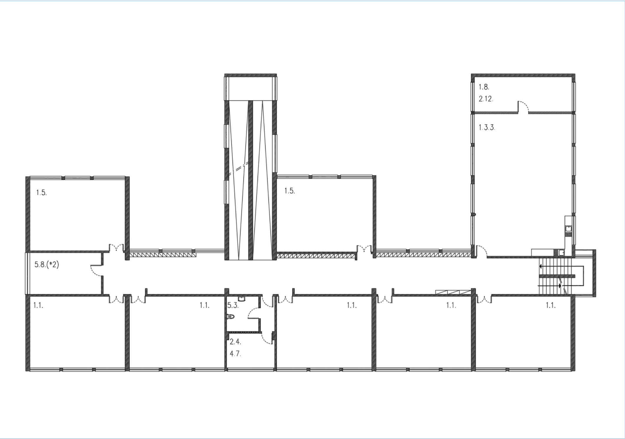
Planta do piso 2
