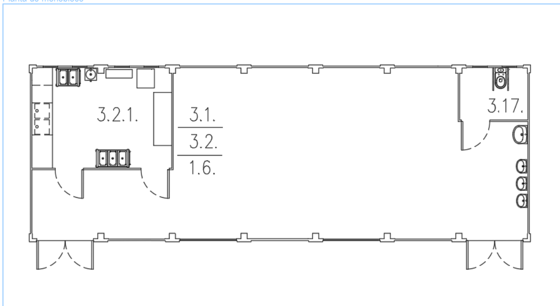
Planta do monobloco
