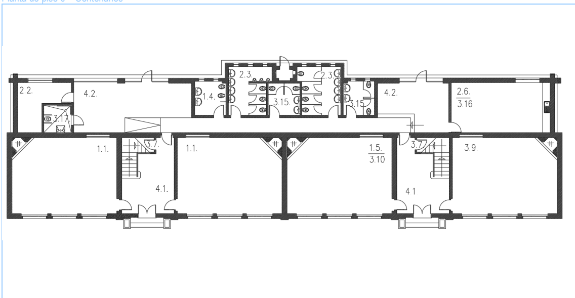
Planta do piso 0 – Centenários
