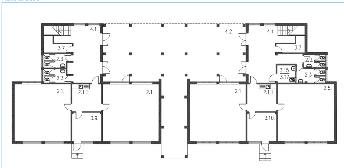
Planta do piso 0
