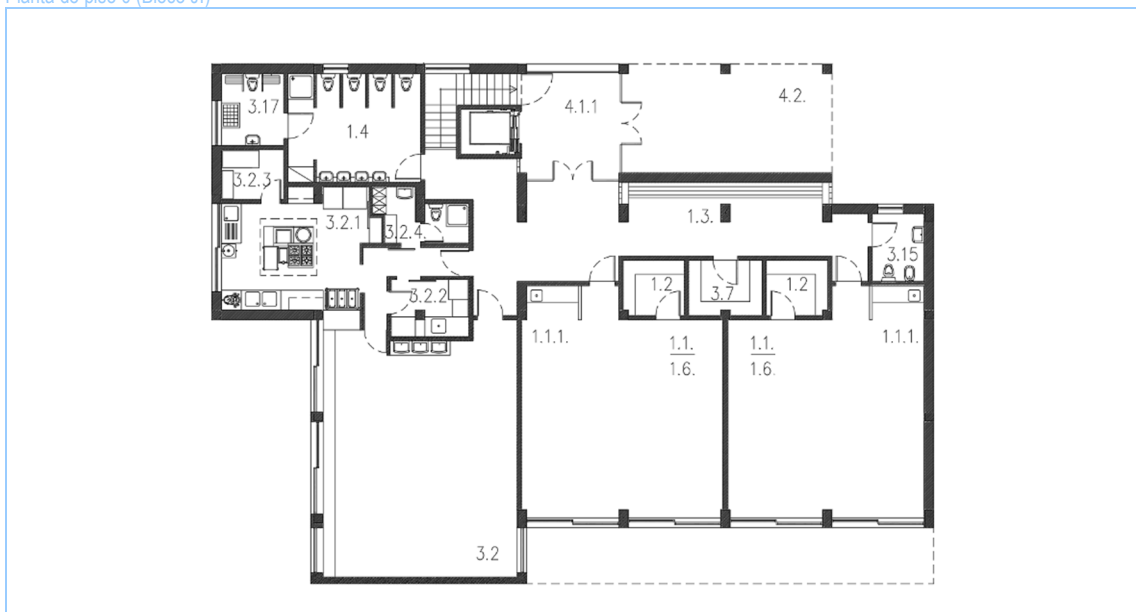
Planta do piso 0 (Bloco JI)
