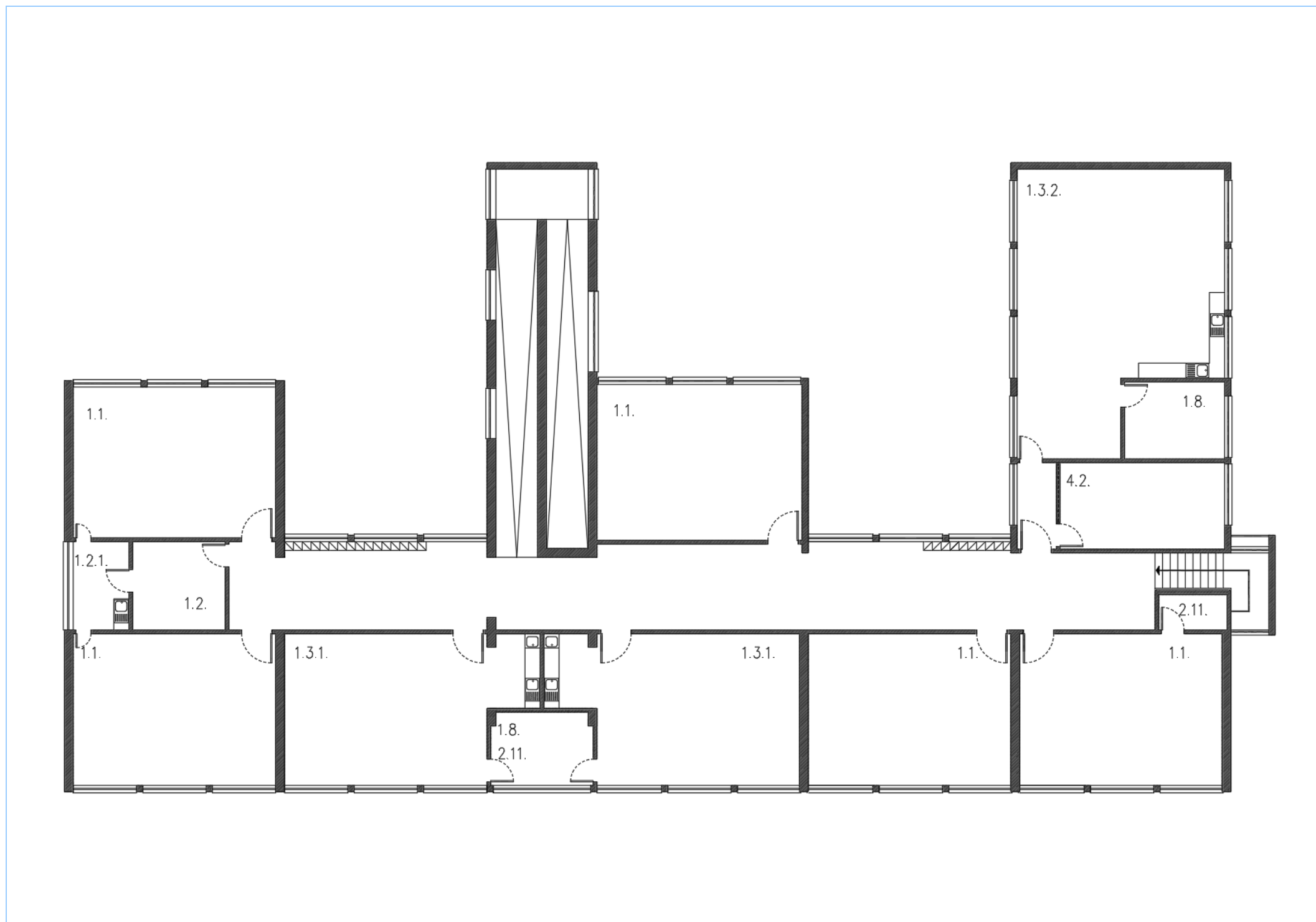
Planta do piso 3
