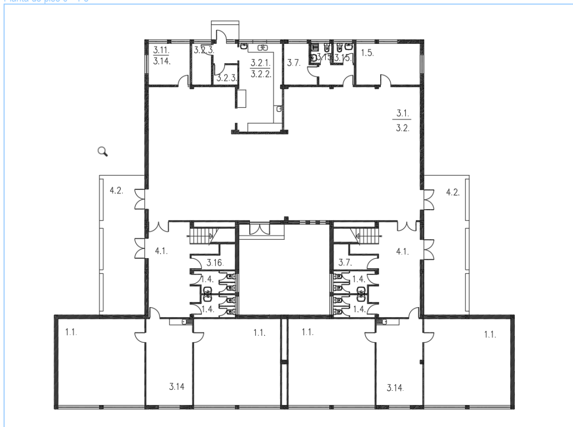
Planta do piso 0 – P3
