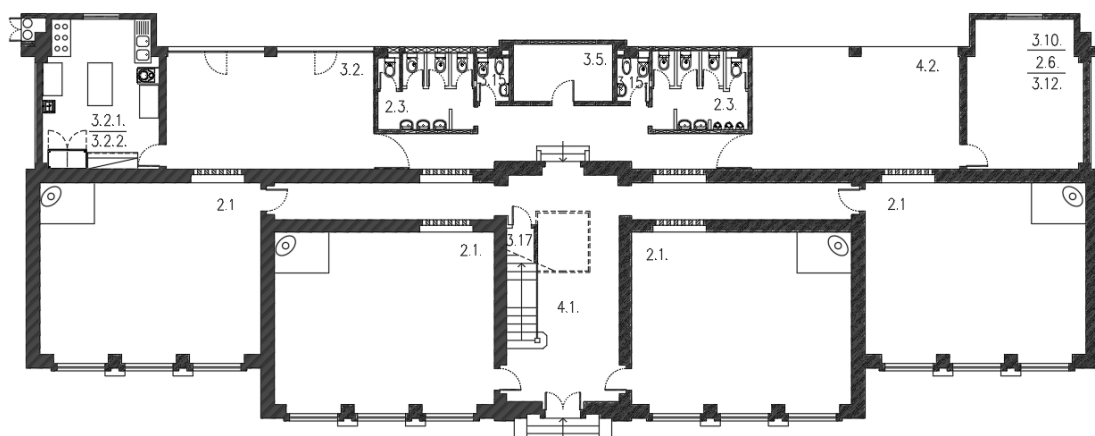
Planta do piso 0
